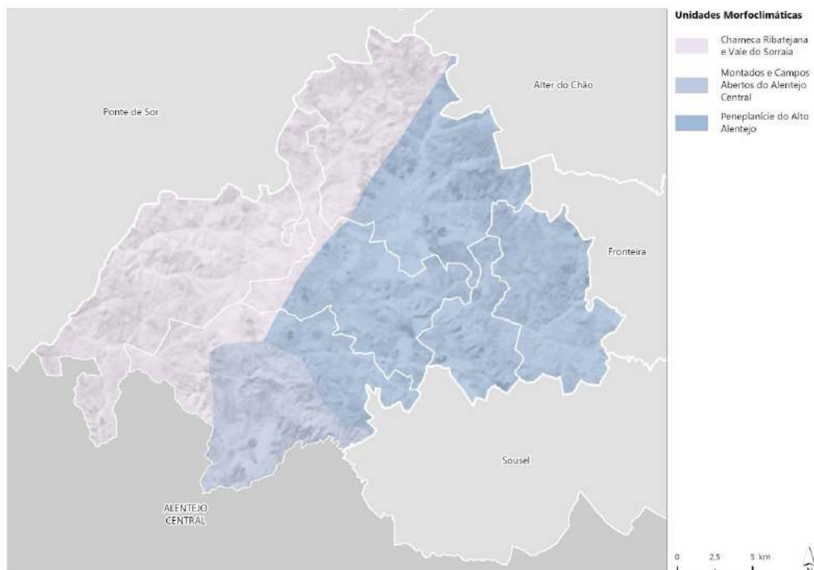
Figura 43. Unidades morfoclimáticas do concelho Fonte: SPI
