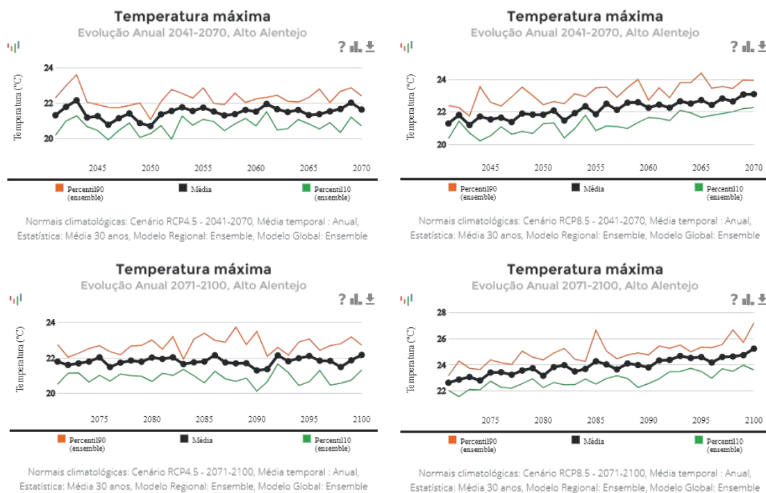
Figura 37. Projeção das anomalias climáticas (médias) da temperatura máxima - para os períodos 2011-2040, 2041-2070 e 2071-2100 - cenário RCP4.5 (à esquerda) e cenário RCP8.5 (à direita)
