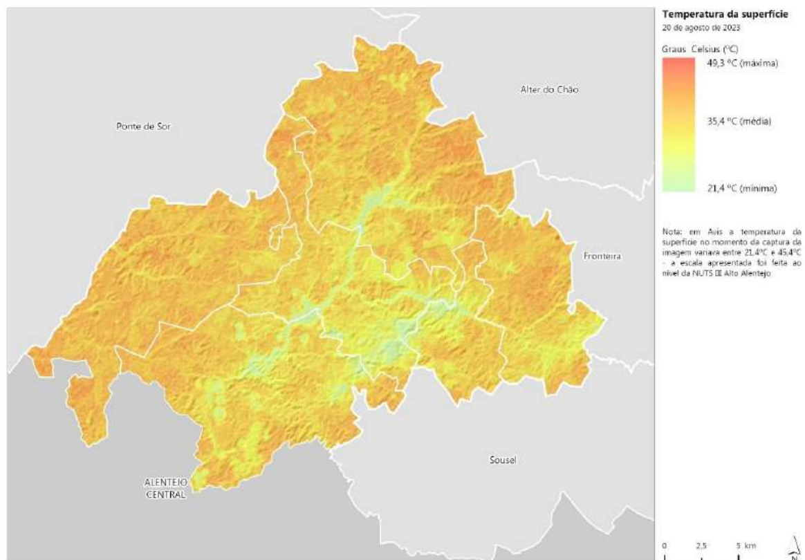
Figura 46. Temperatura da superfície do concelho de Avis em agosto de 2023
