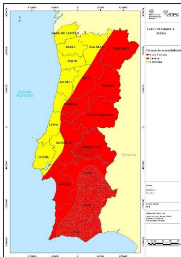
Figura 59. Carta de suscetibilidade a secas Fonte: Adaptado de IPMA apud PROCIV
